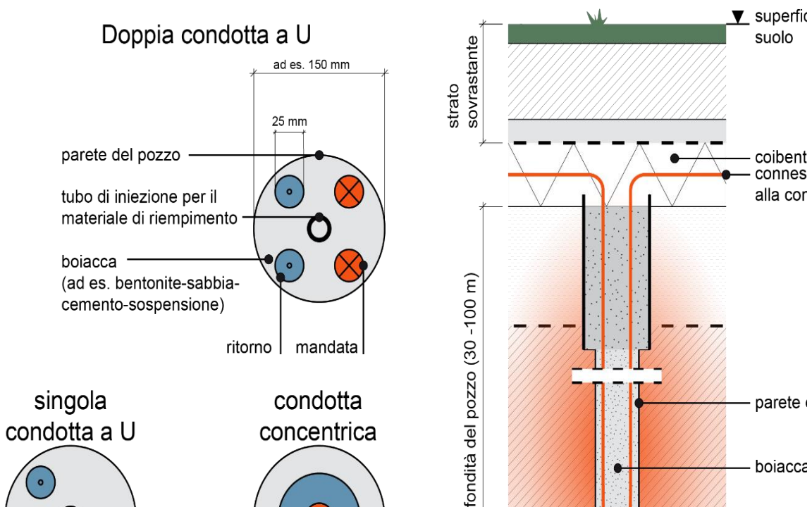
Figura 59: Tipologie comuni e sezione verticale degli scambiatori di calore in pozzo (Fonte: Solites)
