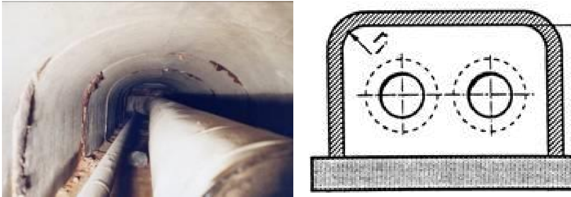
Figura 30: Condotture sotterranee, immagine di un canale rivestito (AGFW, 2013) (sinistra) e un canale rettangolare, come previsto dalla norma DIN 18178 (AGFW, 1993) (destra)
