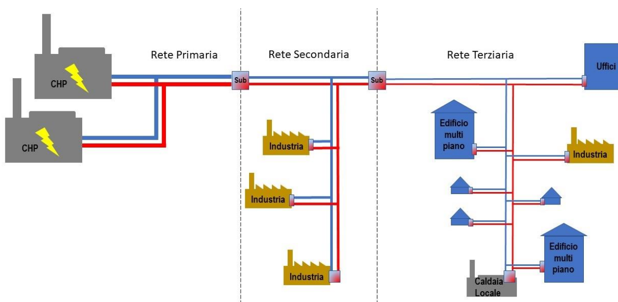
Figura 2: Esempio di rete di teleriscaldamento con una rete primaria, secondaria e terziaria, divisa in sottostazioni, che fornisce calore a diversi tipi di utenti (fonte: D. Rutz)
