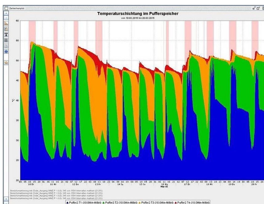
Figura 63: Stratificazione della temperatura nello stoccaggio termico monitorata da Monisoft (Fonte: Hochschule Rosenheim)
