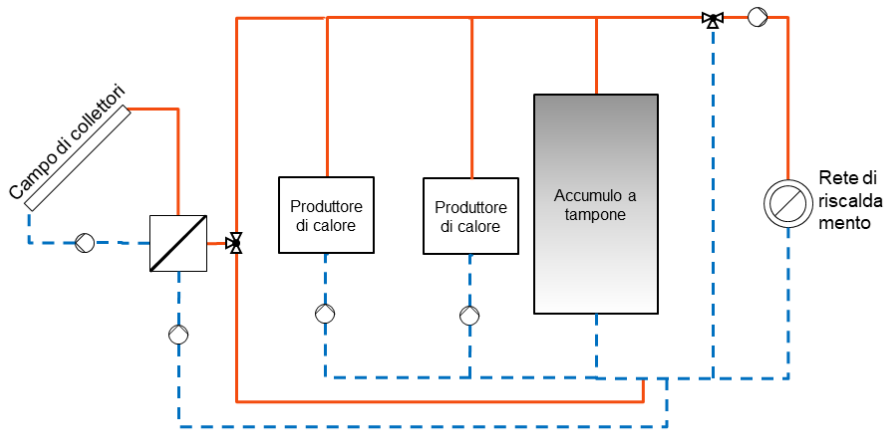
Figura 39: Collegamento in parallelo dei collettori solari termici alla rete di teleriscaldamento e teleraffreddamento per aumentare il flusso di ritorno della rete (Fonte: SOLITES)
