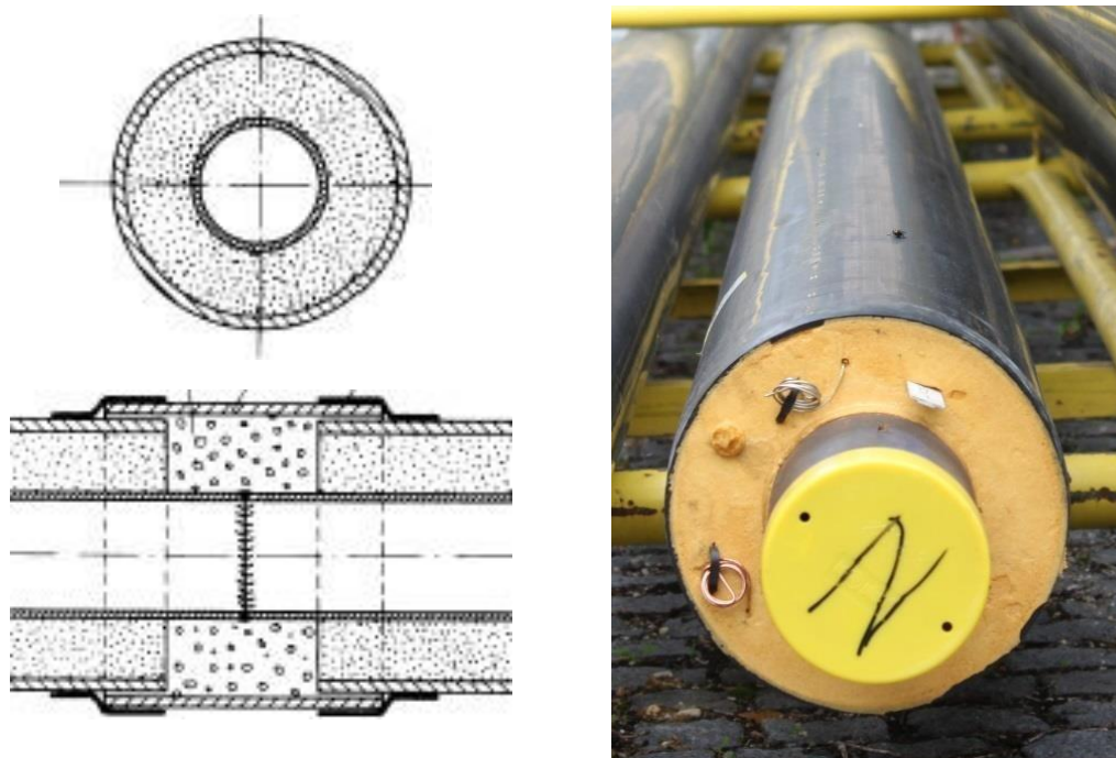
Figura 29: Sezione dei PJP e dei relativi collegamenti (Fonte: AGFW, 1993) (sinistra) e tubature (Fonte: D. Rutz) (destra)
